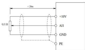
图 3-24 模拟量输入端子接线示意图
