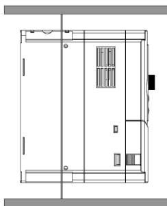
法兰式安装
