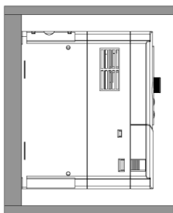
壁挂式安装
