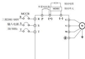
图 3.5 三相 132-315kW
